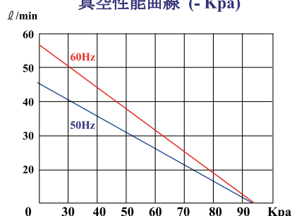
真空性能曲線 (- Kpa)
